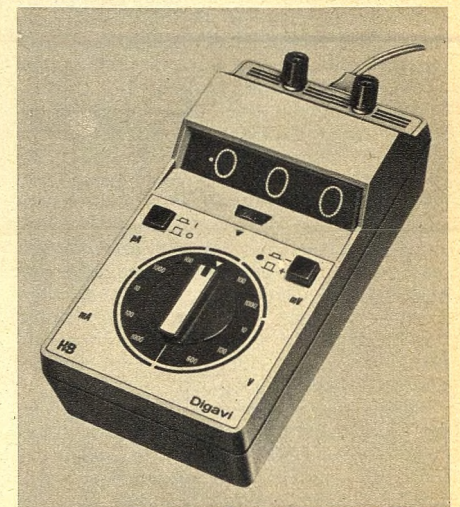
◀ Bild 4. Netzunabhängiges direkt anzeigendes RC-Meter (Mesatronic)
