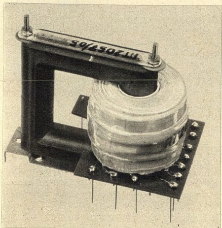
◀ Bild 7. Kombiniertes Horizontalablenk-/Hochspannungstransformator AT 2057/05 von Valvo für die 110°-Eintransformatorenschaltung
