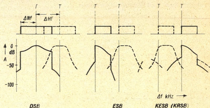
Bild 1. Vergleich von AM-Modulationsarten: DSB = Doppel- oder Zweiseitenbandmodulation, ESB = Einseitenbandmodulation, auch SSB (Single Side Band) genannt, KESB = kompatibles Einseitenbandmodulation, auch KRSB = kompatibles Restseitenbandmodulation genannt. Kanalraster = 9 kHz, Nf-Bandbreite und Empfängerbandbreite = 6 kHz
