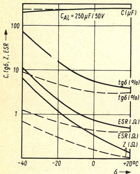
Bild 4. Temperaturverhalten eines Al-Elektrolyt-Kondensators 250 \mu\text{F}/50\text{ V} im Vergleich zwischen wasserhaltigem Glykol-Elektrolyten (Linie) zu einem organischen Elektrolyten (gestrichelt)
