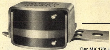
Der MK 1701 ist ein kombinierter Auf- nahme- und Wieder- gabemagnetkopf für das 3,8 mm breite Magnetband. Sein Ein- satz erfolgt in Tonbandgeräten für die Kompakt-
