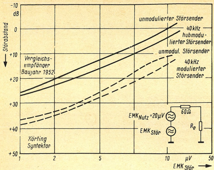
▲ Bild 5. Nachbarkanal Selektion des Syntektors 54 (Messung: RTI)
