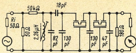
Bild 5. Meßschaltung des Fünfkreis-Hybrid-Keramikfilters der Stemag
