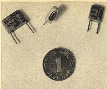
Bild 4. Kunststoffkondensatoren der Baureihen FKS 2 und FK 2. Zu beachten bei dem Schnitt in der Mitte ist die geringe Wandstärke. Der rechte Kondensator hat das Rastermaß 5 (Aufnahme: Schwahn)
