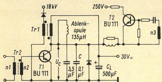
Bild 1. Vereinfachte Horizontal-Ablenkung nach dem Pump-Konzept
