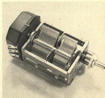
Bild 1. Abstimmpotentiometer, angebaut an einen AM-Drehkondensator, der Karl Hopt GmbH (Aufnahme: Schwahn)
