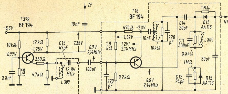
Bild 6. Schaltung des Syntro-Detektors mit Transistoren im Jahre 1969/70 (Körting-Hi-Fi-Steuergerät Syntector 1500 L)
